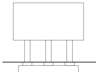
【3本柱1基礎】
